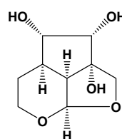
picrococin D
