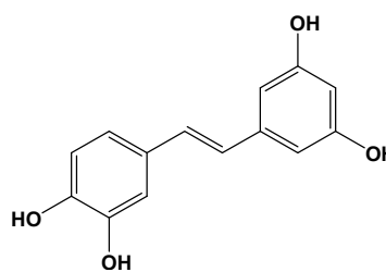
piceatannol
