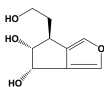
picrococin A
