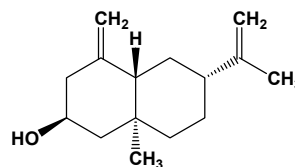
jatamol A
