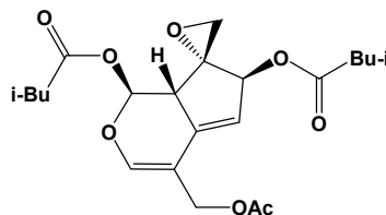
valtrate
