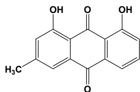
chrysophanol
