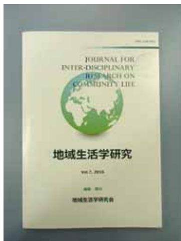
図 4-24 学術雑誌
