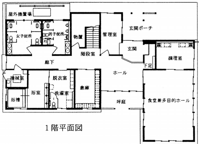
▲ 「ゆうゆう館」平面図
