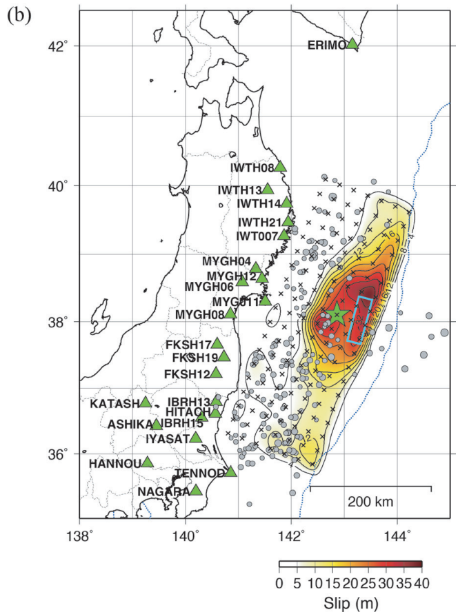
第 1.4.5 図 近地強震記録を使った震源過程解析結果 (a) モーメントレート関数. (b) 断層面上のすべり分布. 星印は震源(破壊開始点)の位置, 丸印は本震発生後1日以内に起きたM5以上の余震. ×印は仮定した小断層の中心位置, 三角は解析に使用した観測点を示す. すべり量のコンターは4mごとである. 水色の長方形は津波波形記録より求めた海底が大きく隆起した領域 (Hayashi et al. , 2011).
