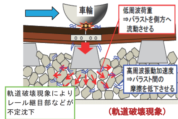
図2 バラスト軌道の不定沈下
